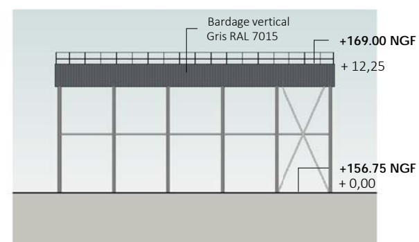
③ Façade Est 1 : 500
