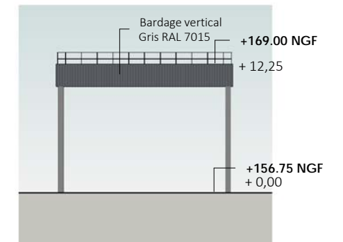
⑥ Façade Sud 1 : 500
