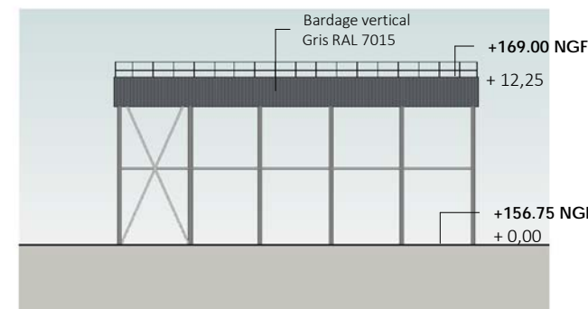
⑤ Façade Ouest 1 : 500
